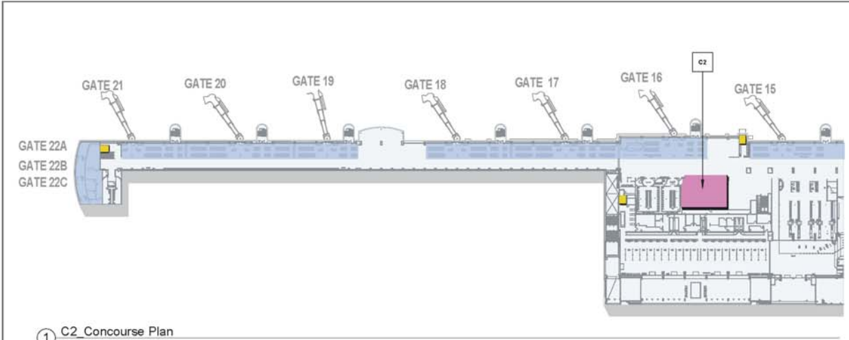
① C2 Concourse Plan N.T.S.
