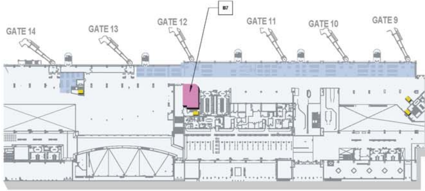
① B7 Concourse Plan N.T.S.
