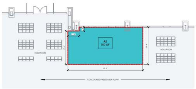
② A2 1/16" = 1'-0"
